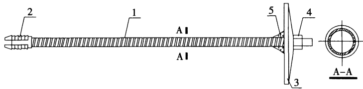
图 A.0.4 钢质涨壳中空注浆锚杆
