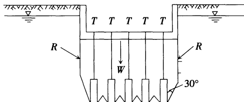
图 1 考虑群锚效应的锚杆抗浮作用
