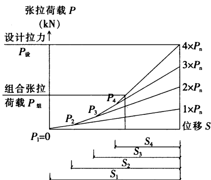
图 10 张拉管理
