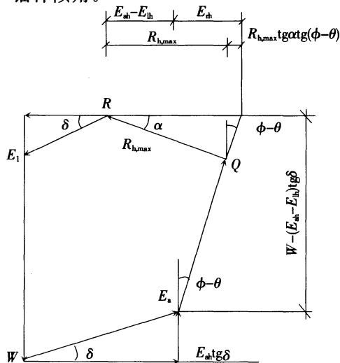
图 7 力多边形几何关系
