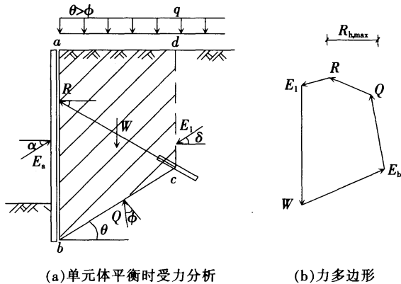
图 6 锚杆沿深层滑动面稳定性验算
