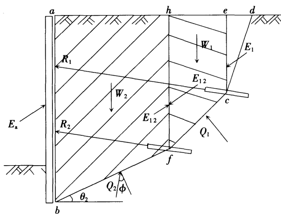
(b) 力系平衡
