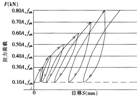
图 E. 0.1 锚杆基本试验荷载-位移曲线
