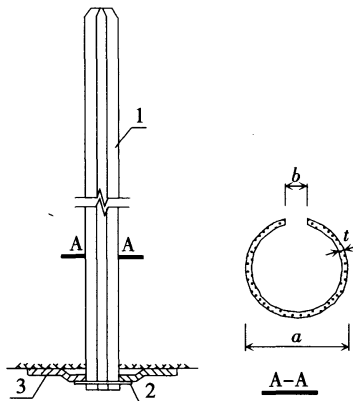
图 A.0.5 缝管锚杆
