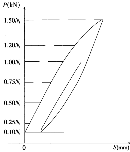
图 F 锚杆荷载-位移曲线
