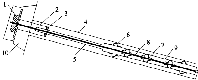
图 6.2.1-1 锚杆Ⅰ级防护构造
