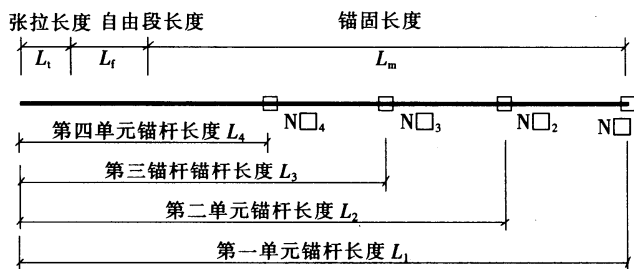
图 9 荷载分散型锚杆长度示意
