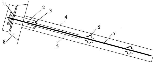
图 6.2.1-2 锚杆Ⅱ级防护构造
