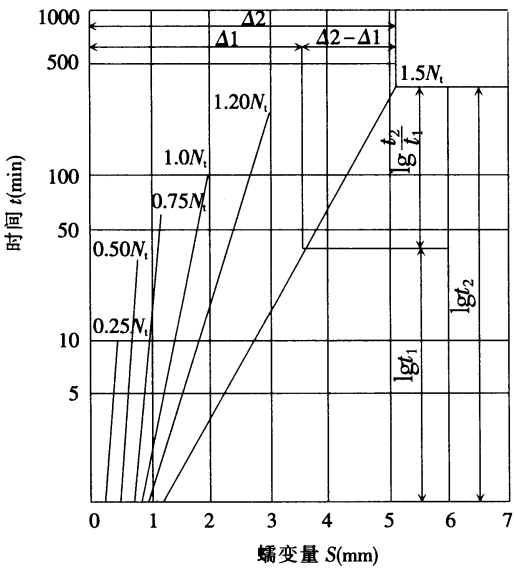
图 G 锚杆蠕变量-时间对数曲线
