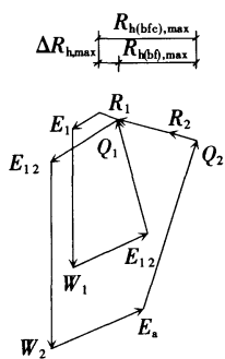
(c) 力多边形几何关系
