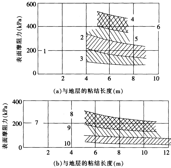
图 4 用与不用二次注浆的锚杆随锚固长度变化的实测表面摩阻力 1—中等塑性粘土;2—不进行二次注浆的很硬粘土;3—不进行二次注浆的硬粘土; 4—进行二次注浆的硬至极硬的粘土;5—不进行二次注浆的硬至极硬粘土; 6—中等塑性的砂质粉土;7—中到高塑性粘土;8—进行二次注浆的极硬粘土; 9—不进行二次注浆的极硬粘土;10—不进行二次注浆的硬粘土
